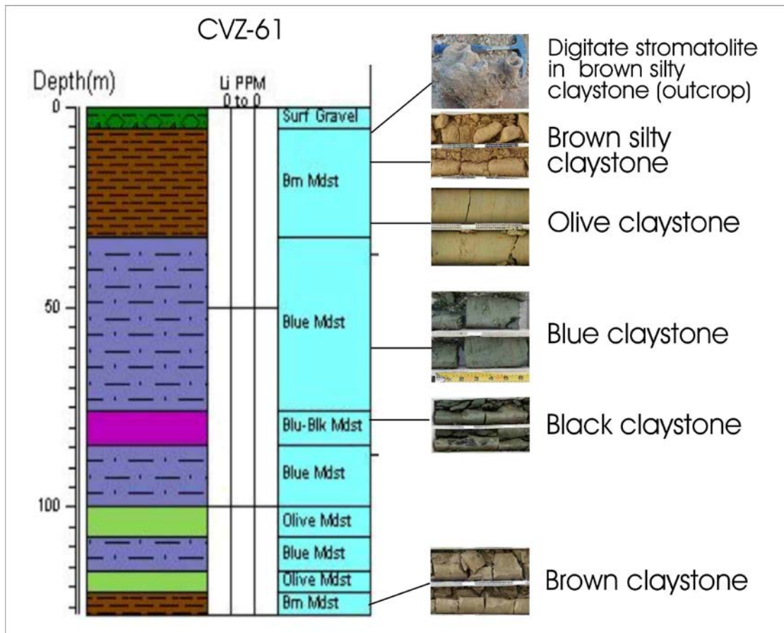
Abb. 1: Stratigrafie und Kernfotos von Bohrloch CVZ-61. Dieses Bohrloch enthält 91 Meter mit Lithium-Tonstein in Einheiten von variabler Farbe. Alle Tonsteineinheiten mit Ausnahme des braunen verschlammten Tonsteins weisen relativ hohe Lithiumkonzentrationen in früheren Bohrlöchern im Konzessionsgebiet auf.
